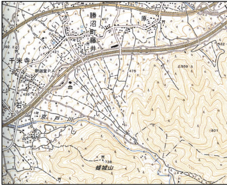
8 図 山梨県石和町の地形図
